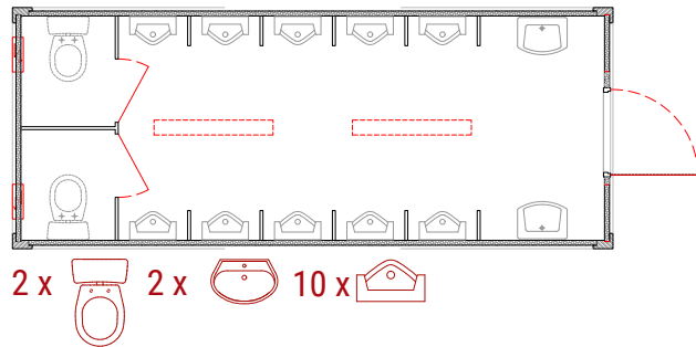
Container sanitaire Type 20' - Maxi WC 6055 x 2435 x 2591
